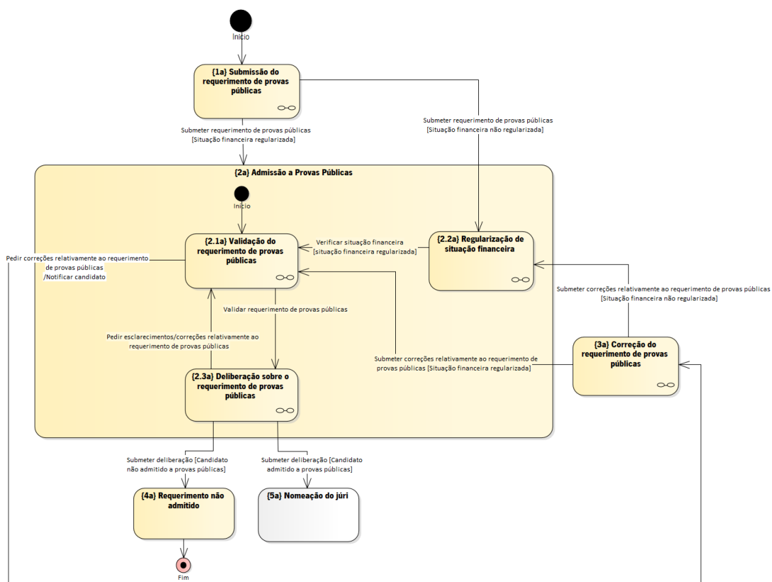
Figura 1: Desmaterialização do processo de provas públicas conducentes ao grau de Mestre (em UML).
