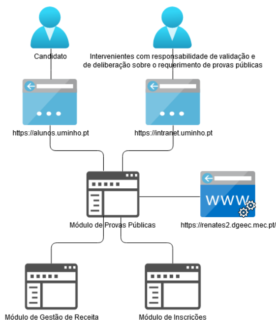
Figura 13: Módulos e plataformas informáticos envolvidas na desmaterialização do processo de provas públicas.
