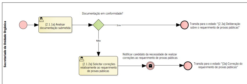
Figura 3: Validação do requerimento de provas públicas - grau de Mestre (em BPMN).
