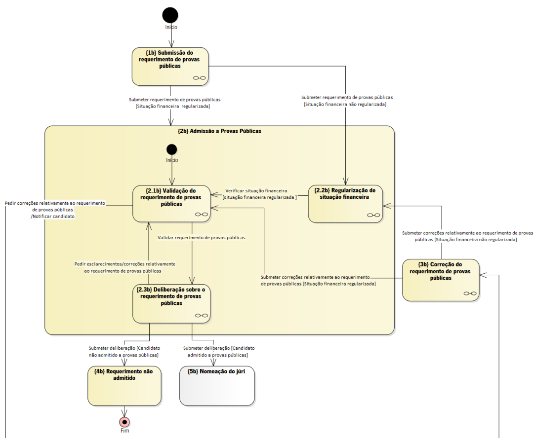
Figura 7: Desmaterialização do processo de provas públicas conducentes ao grau de Doutor (em UML).
