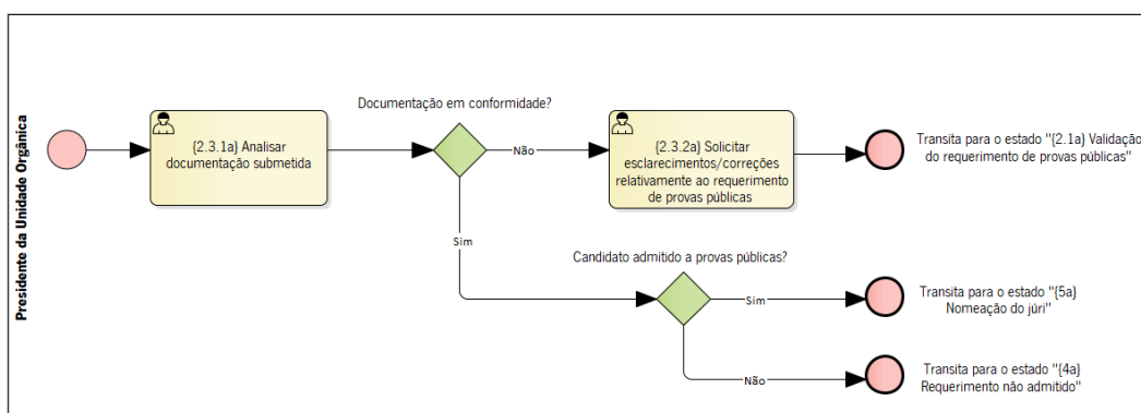
Figura 5: Deliberação sobre o requerimento de provas públicas - grau de Mestre (em BPMN).
