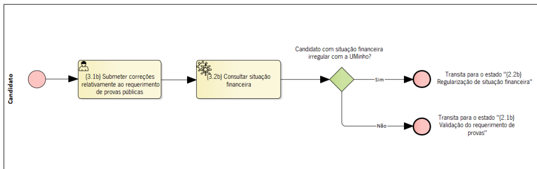
Figura 12: Correção do requerimento de provas públicas - grau de Doutor (em BPMN).
