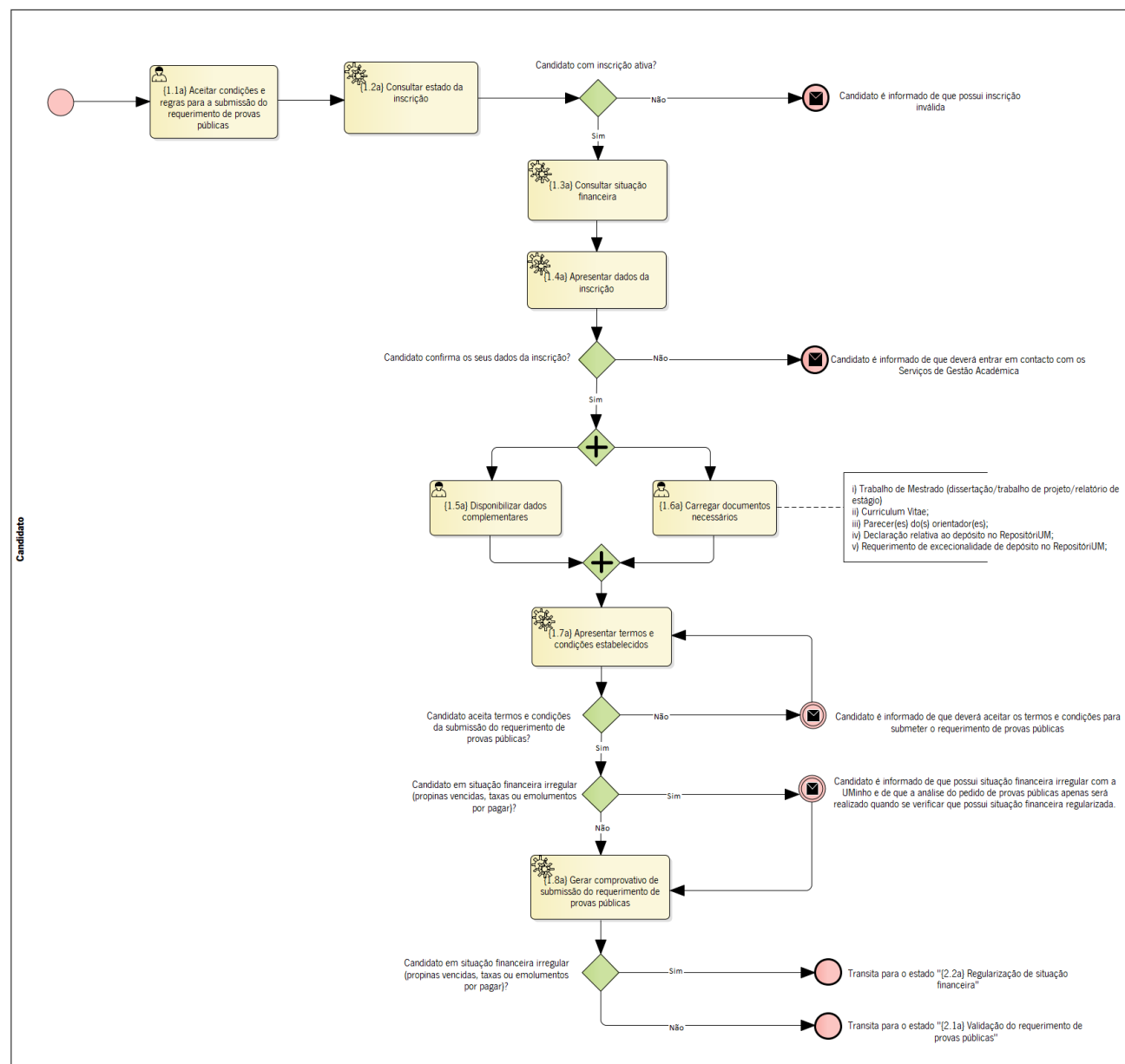
Figura 2: Submissão do requerimento de provas públicas - grau de Mestre (em BPMN).
