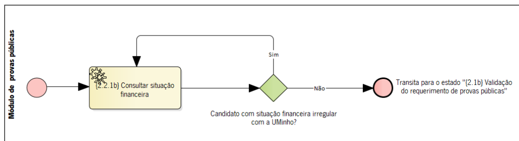
Figura 10: Regularização de situação financeira - grau de Doutor (em BPMN).
