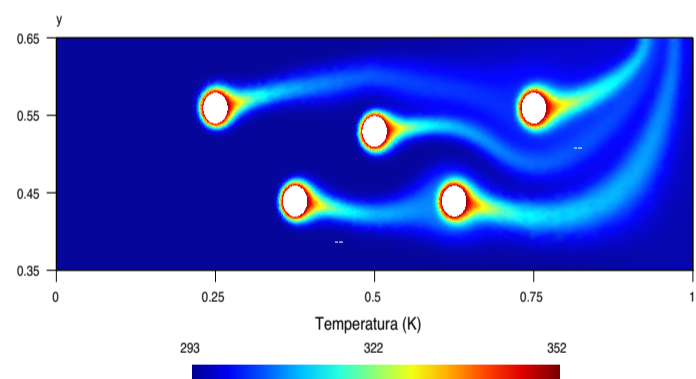
Resultado da simulação onde se evidenciam as temperaturas e as trocas energéticas no refrigerador
