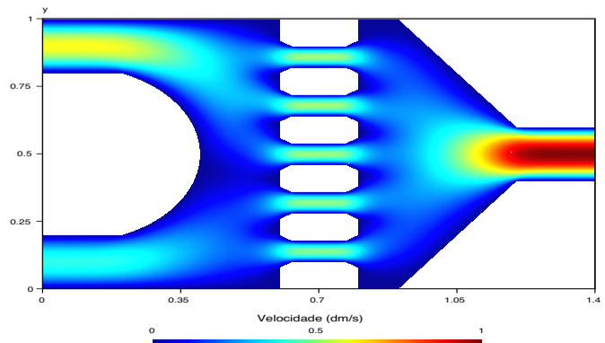
Resultado da simulação onde se evidenciam as velocidades do polímero no interior da extrusora.
