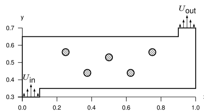
Representação esquemática de um refrigerador.
